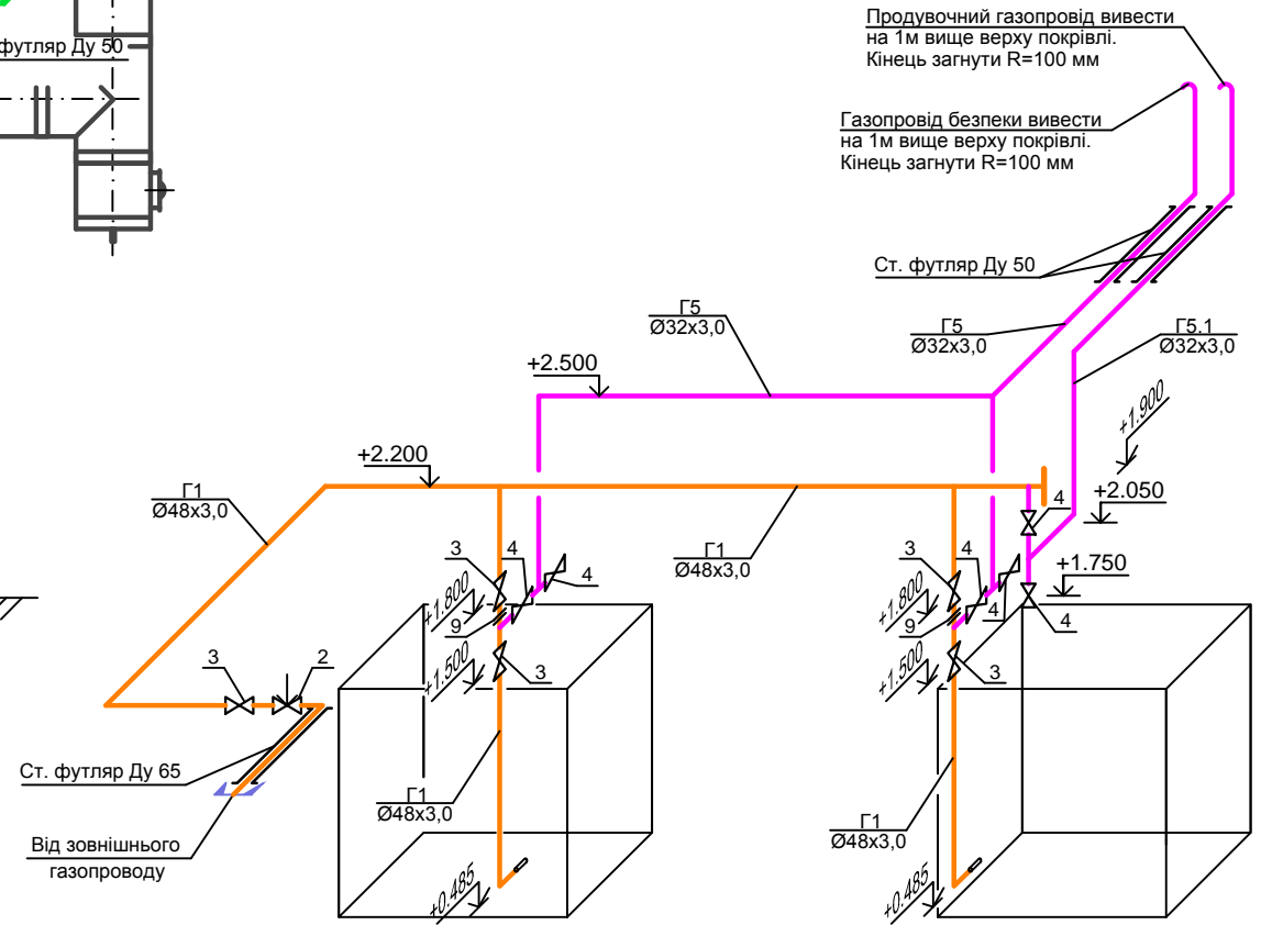
АксонOMETрична схема
