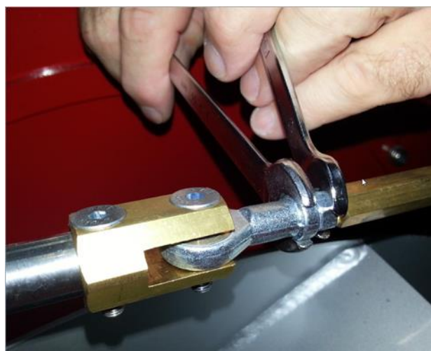
Fig. 46 для регулировки ослабить контргайку
