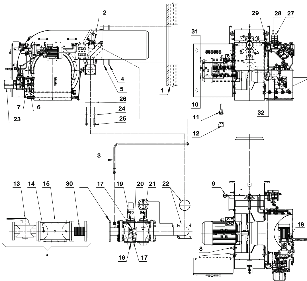
Fig. 4 УСТАНОВКА ГОРЕЛКИ
