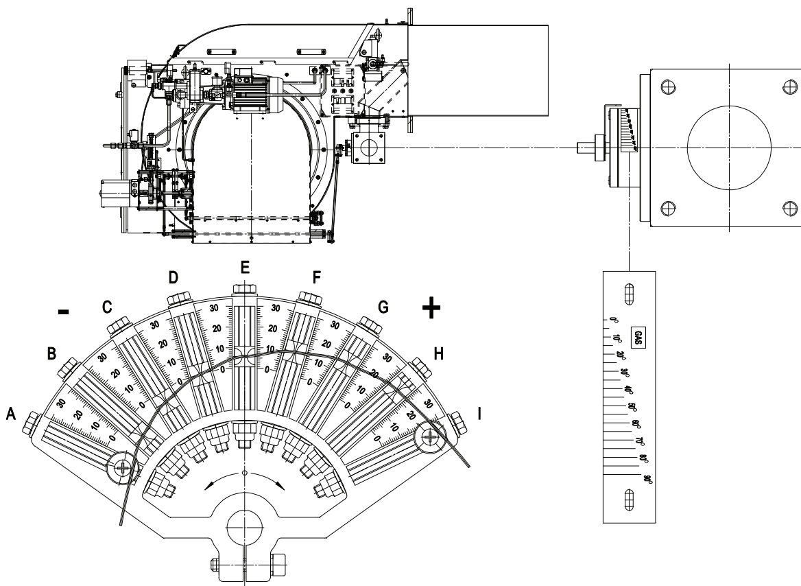
Fig. 27 ГАЗОВЫЕ ЭКСЦЕНТРИКИ
