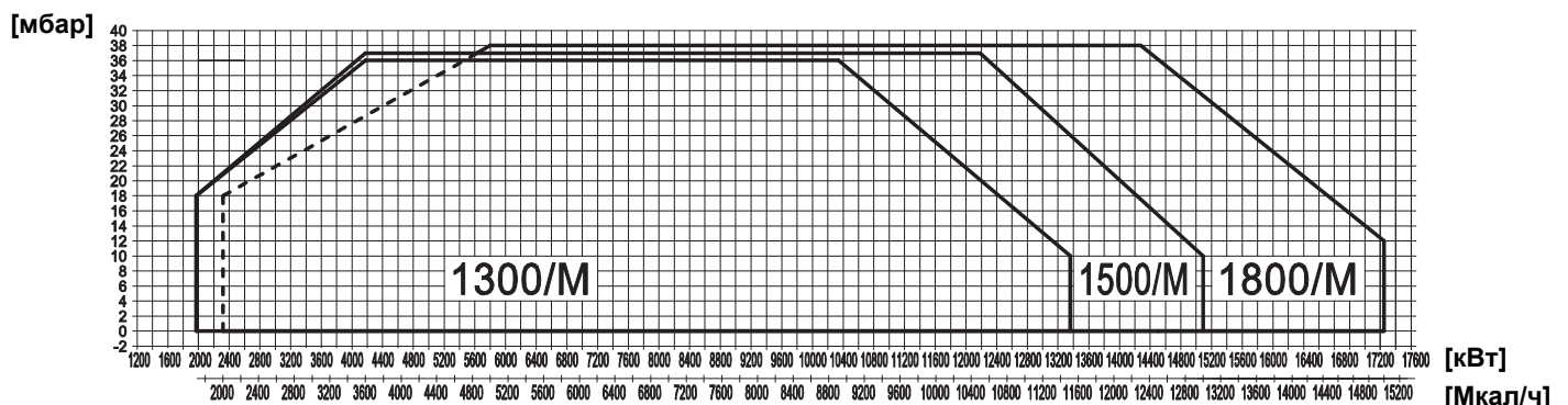
Fig. 2 X = Мощность Y = Соппротивление камеры сгорания
